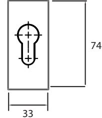
Square Escutcheon
